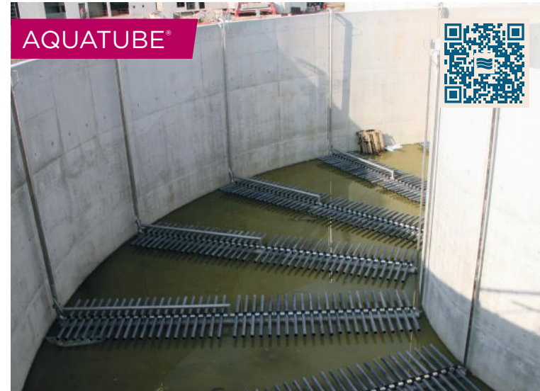
AÉRATION DES BASSINS À BOUES ACTIVÉES DE STEP URBAINES ET INDUSTRIELLES
